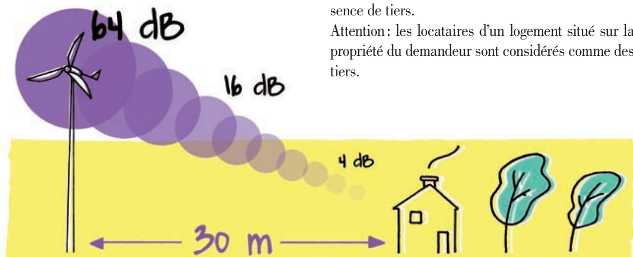
LE BRUIT DÉCROÎT FORTEMENT AVEC LA DISTANCE : SELON UN FACTEUR 4 À UNE QUINZAINE DE MÈTRES, ET UN FACTEUR 8 À UNE TRENTAINE DE MÈTRES.
