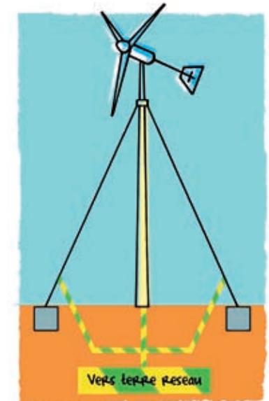
LA MISE À LA TERRE SE FAIT PAR DE LA CABLETTE DE FILS DE CUIVRE NUS INTERCONNECTÉS.
