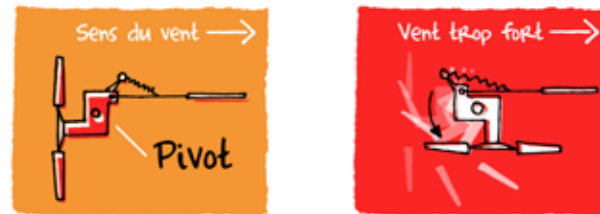
PRINCIPE DE L'EFFACEMENT, APPELÉ AUSSI "FURLING", ICI LATÉRAL.
